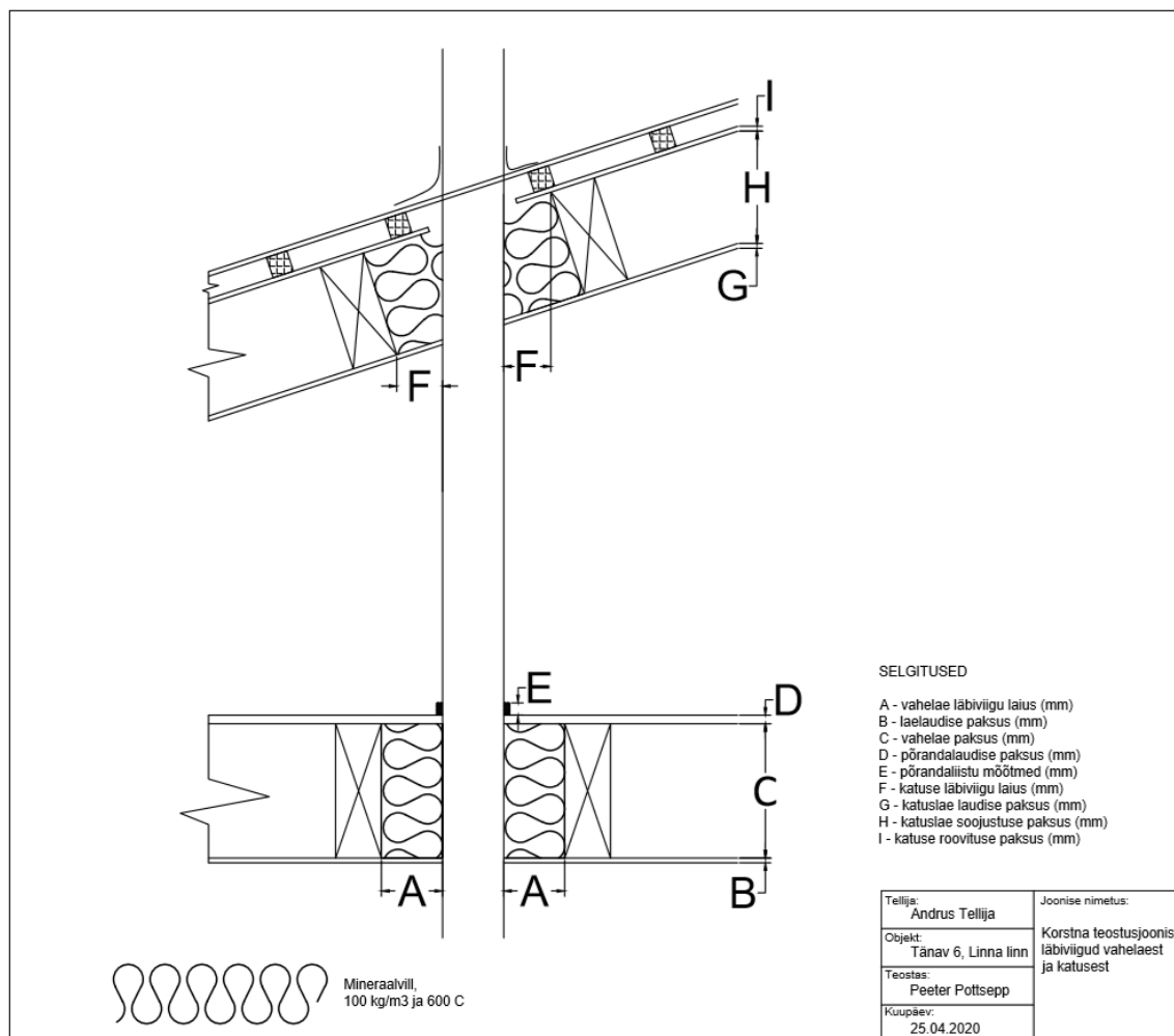
Korstna läbiviigu teostusjoonise näidis
