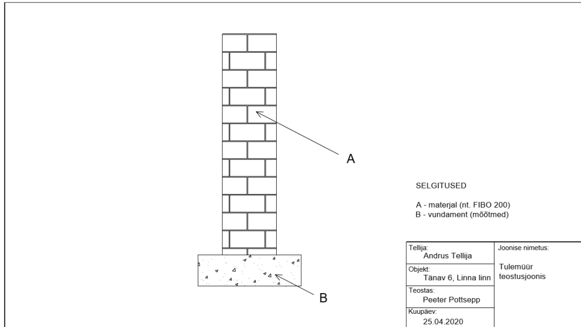
Tulemüüri teostusjoonis
