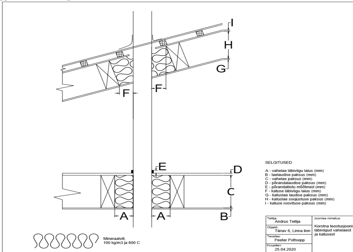
Joonis 5 Korstna läbiviigu teostusjoonise näidis
