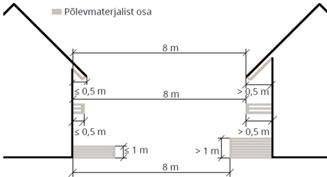
Joonis 1 Hoonete vaheline ohutu vahekaugus
